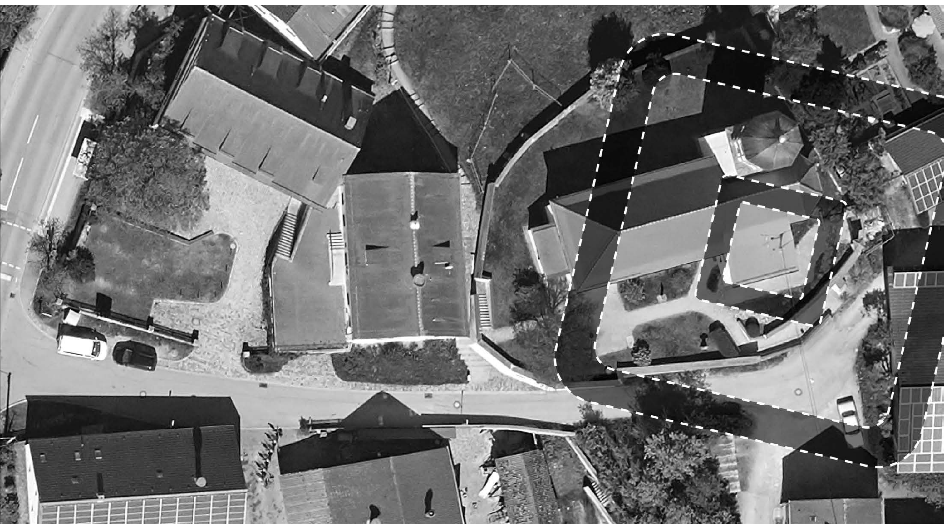
Luftbild 2019 und Grundriß des spätrömischen Wachturmes mit Umwallung, Finningen (Stadt Neu-Ulm, Stefan Reuter)
